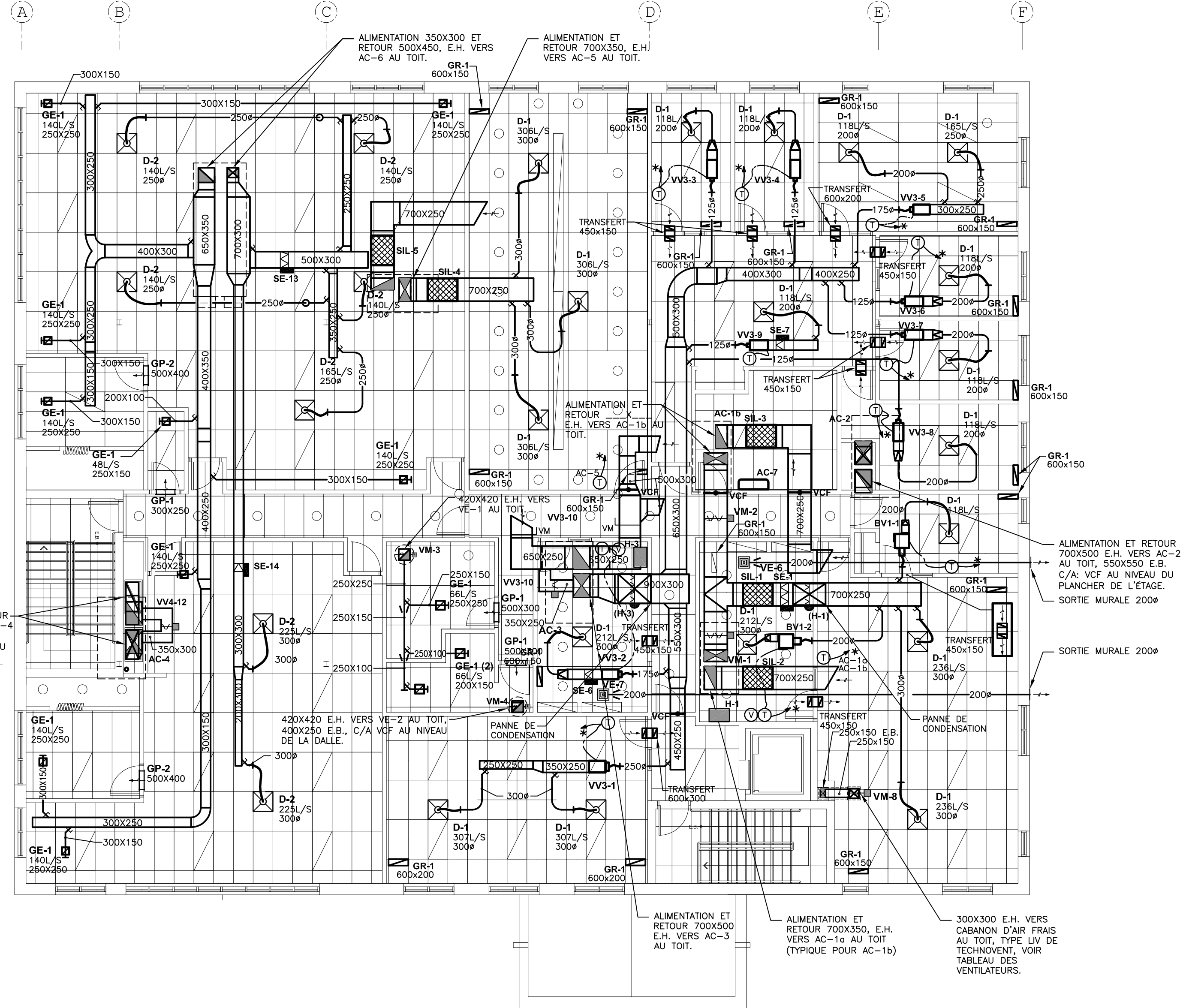
PLAN DE L'ÉTAGE
