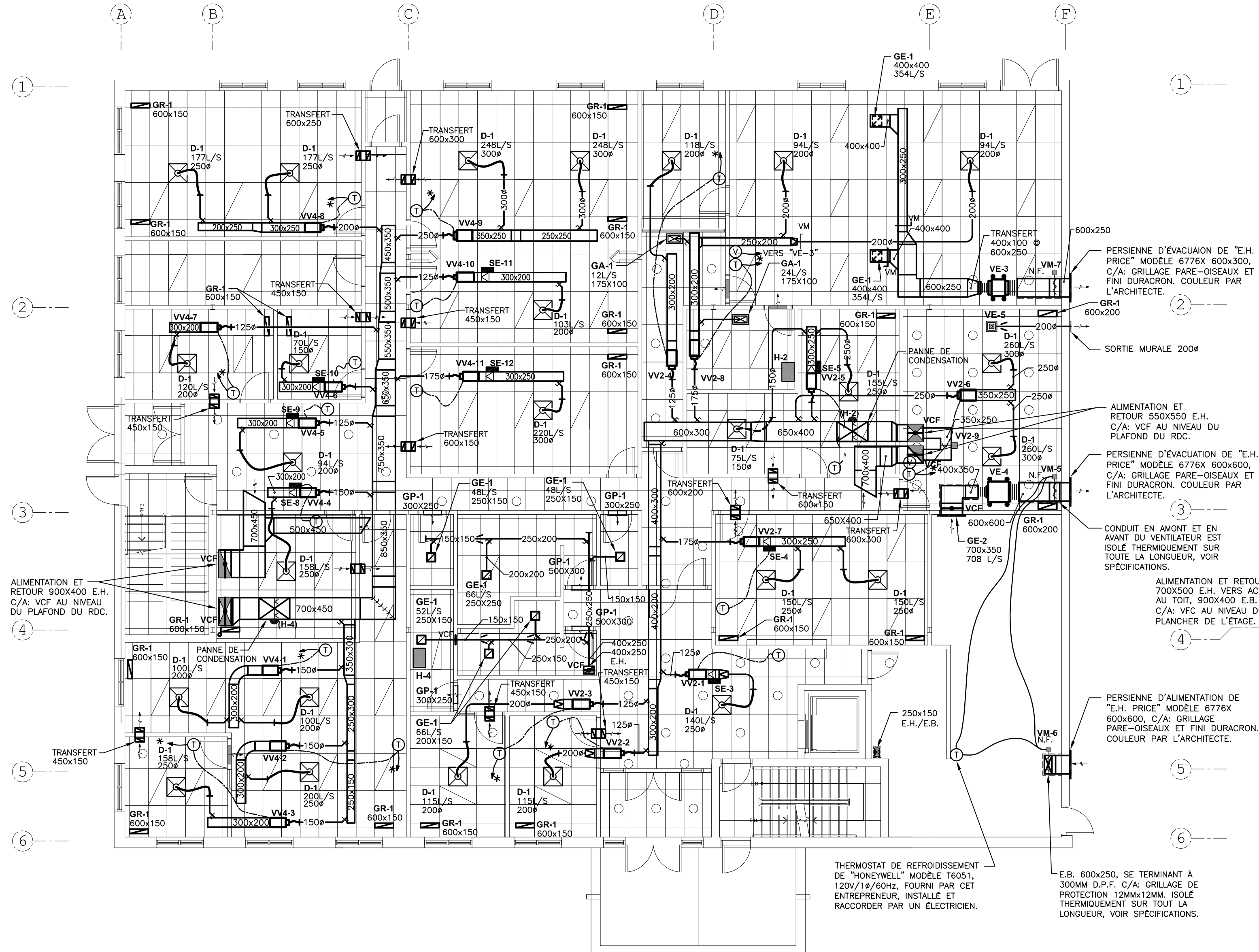
PLAN DU REZ-DE-CHAUSSÉE
