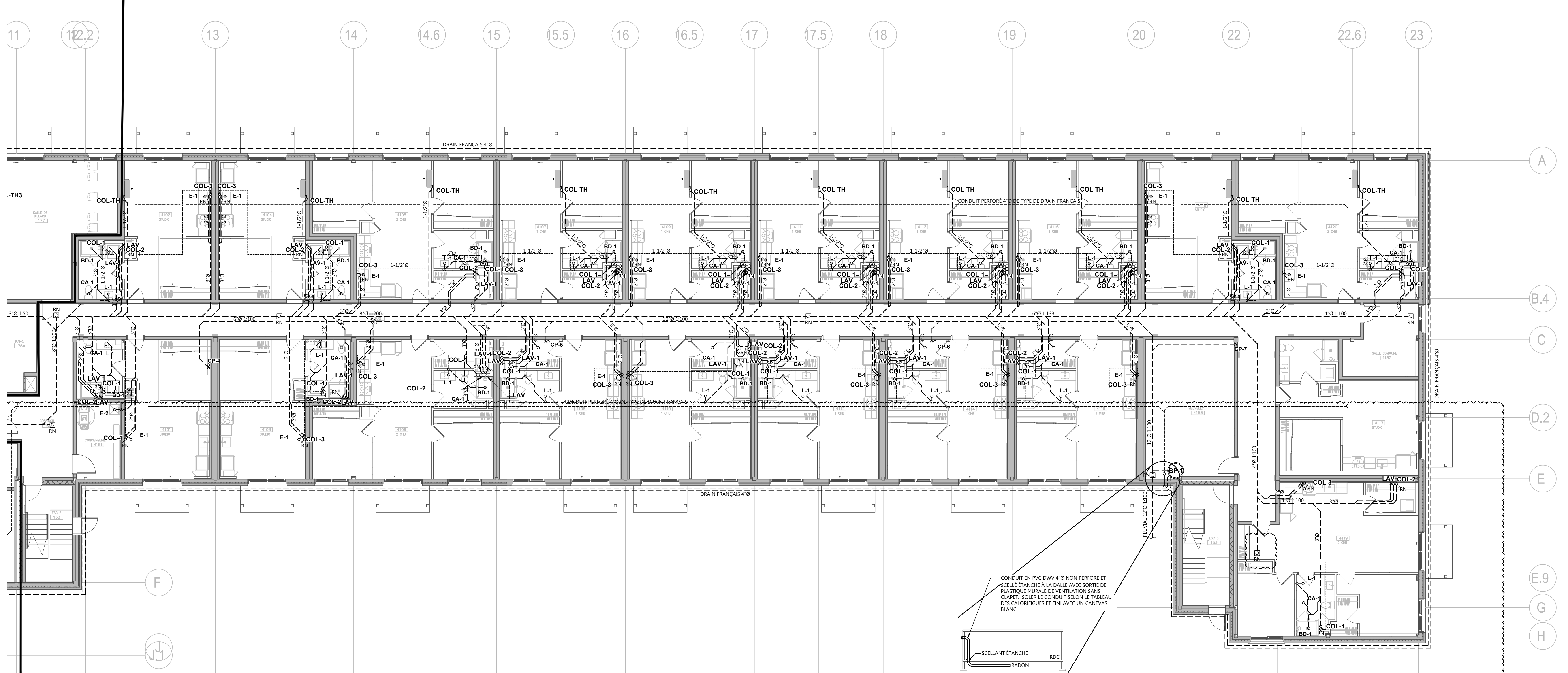
PLAN D'AMÉNAGEMENT DRAINAGE : NIVEAU 1 PARTIE DROITE ÉCHELLE : 1/8" = 1'-0"
